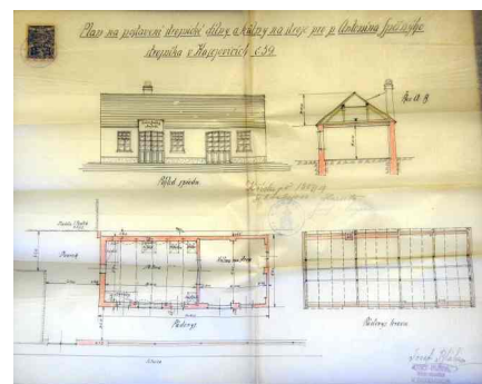
Plán na výstavbu strojnické dílny se skladem pro Antonína Spěšného v Kasejovicích roku 1919 (SOkA Plzeň-jih se sídlem v Blovicích, AM Kasejovice, inv. č. 767, kart. 96).
